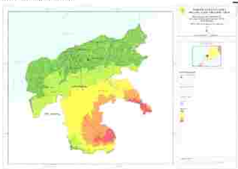
Gambar II.2 Peta Ketinggian Lahan
